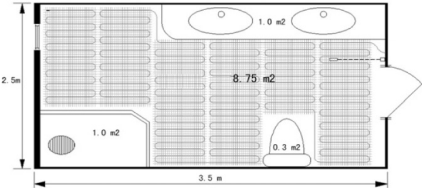
2. ábra – a fűtőfelület kiszámítása
