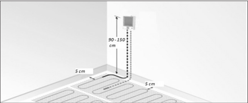
3. ábra – jellemző bekötési vázrajz
